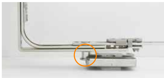
Höhenverstellbarer Pilzkopfzapfen und Sicherheitsschliessblech
